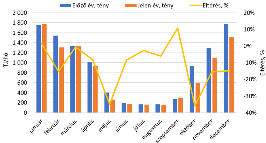
6. ábra: Értékesített hőmennyiség
