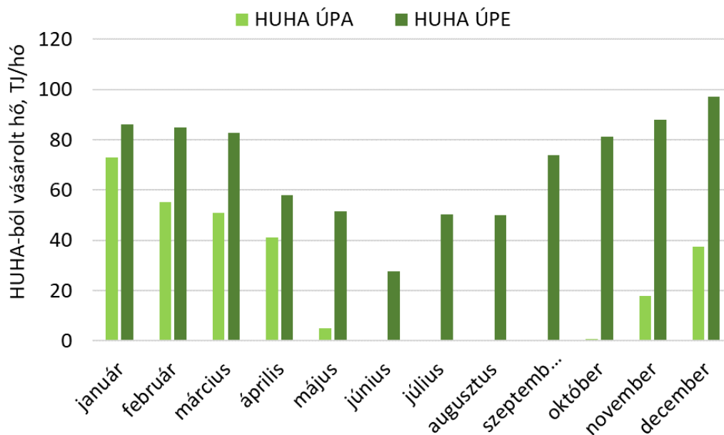
12. ábra: 2022. évben megvalósított hőkooperáció
