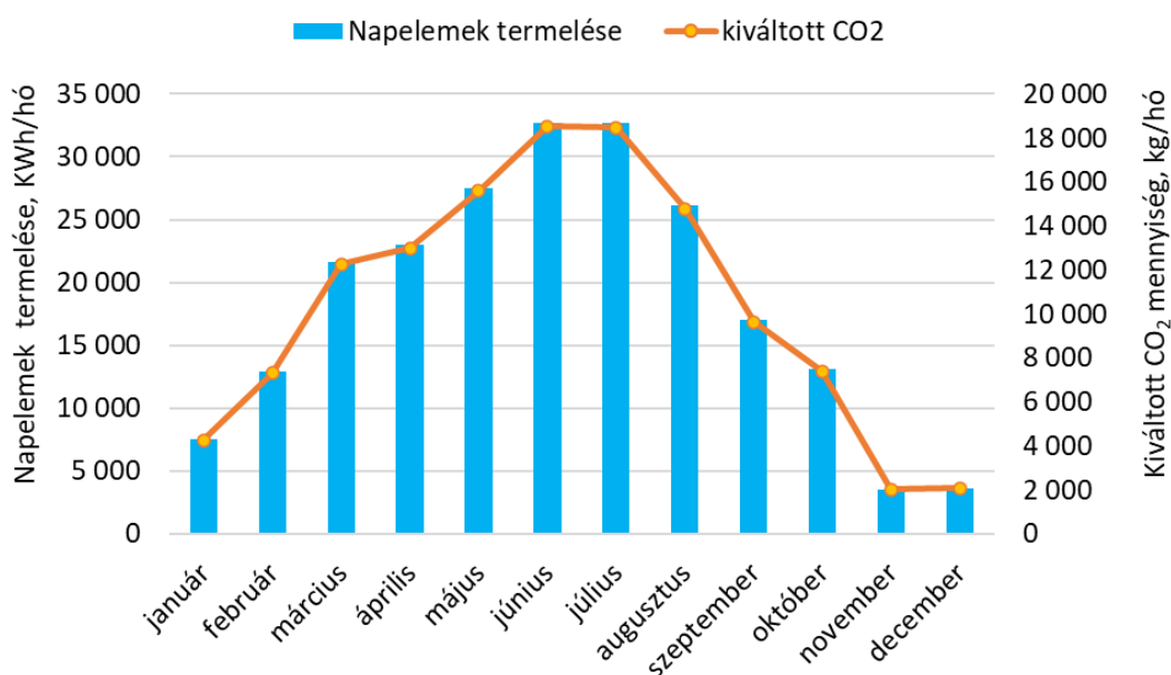
11. ábra: Napelemek 2022. évi villamosenergia-termelése
