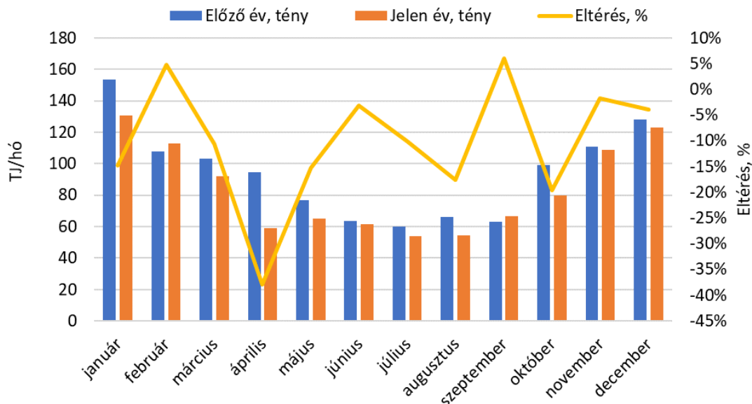
7. ábra: Távhőköri veszteség alakulása
