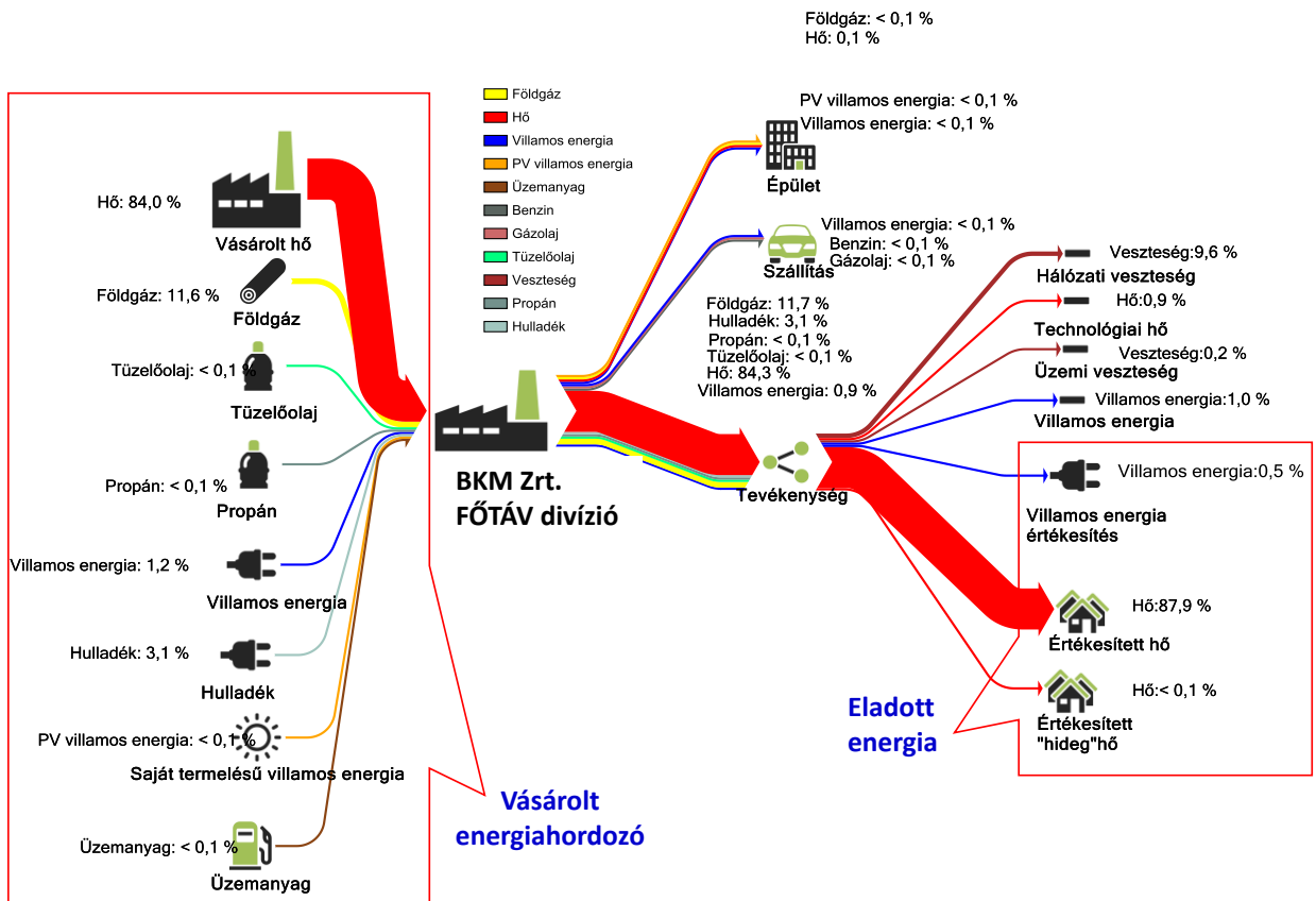
2. ábra: A FŐTÁV Zrt. 2021. évről való adatszolgáltatás energiafolyam ábra
