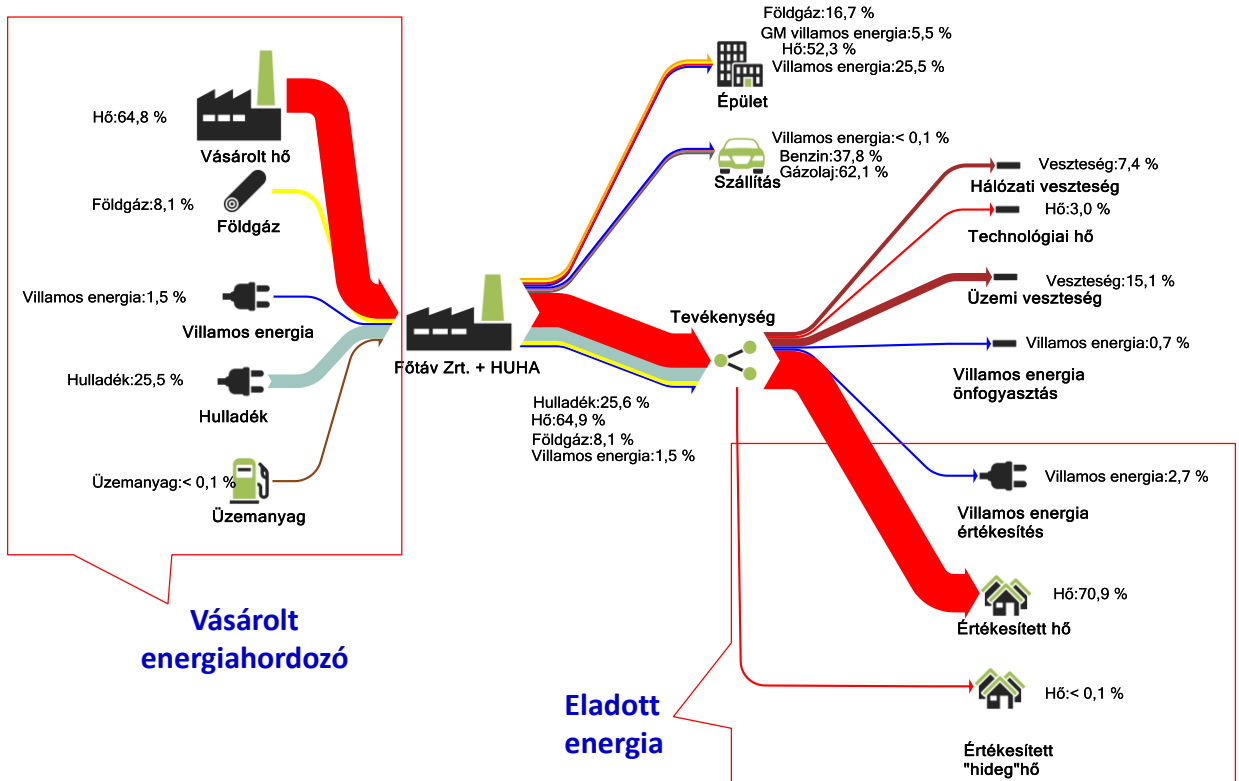
3. ábra: A BKM Nonprofit Zrt. FŐTÁV divízió 2022. évi energiafolyam ábrája
