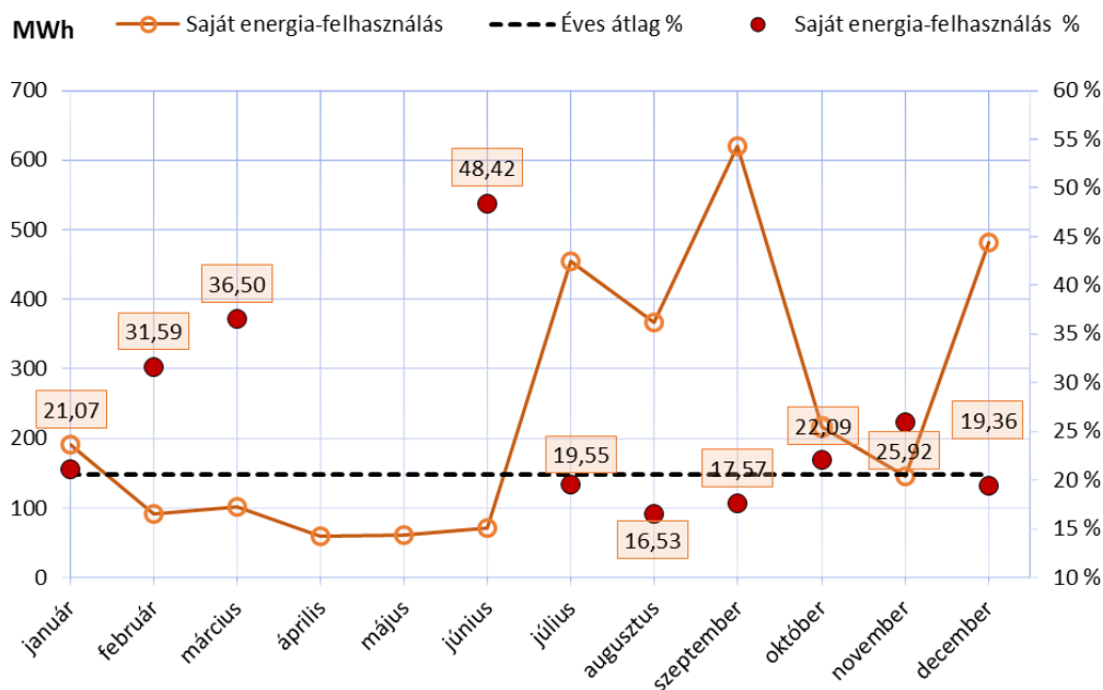
9. ábra: Saját hatáskörbe eső energiafogyasztás elemzése
