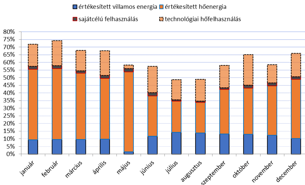
10. ábra: Hasznos energiák megoszlása a kazánok által megtermelt gőzenergia függvényében
